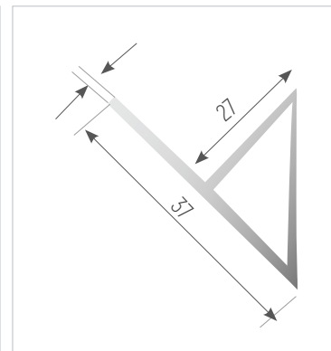
Berenjeno ala Large chamfer strip Liteau triangulaire avec aile
